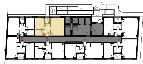
prizemna etaža
